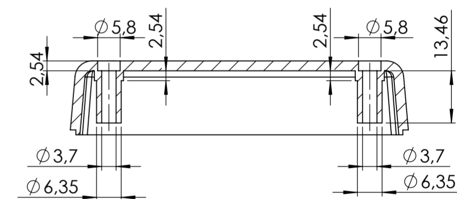
SEZIONE B-B
