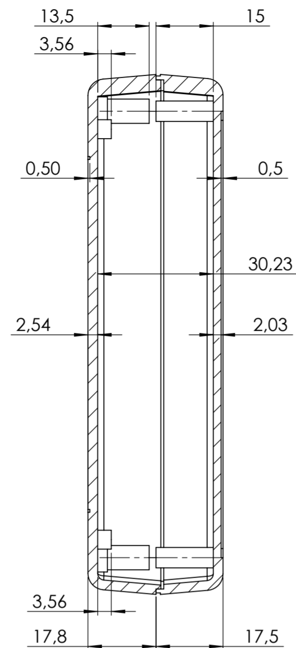
SEZIONE A-A
