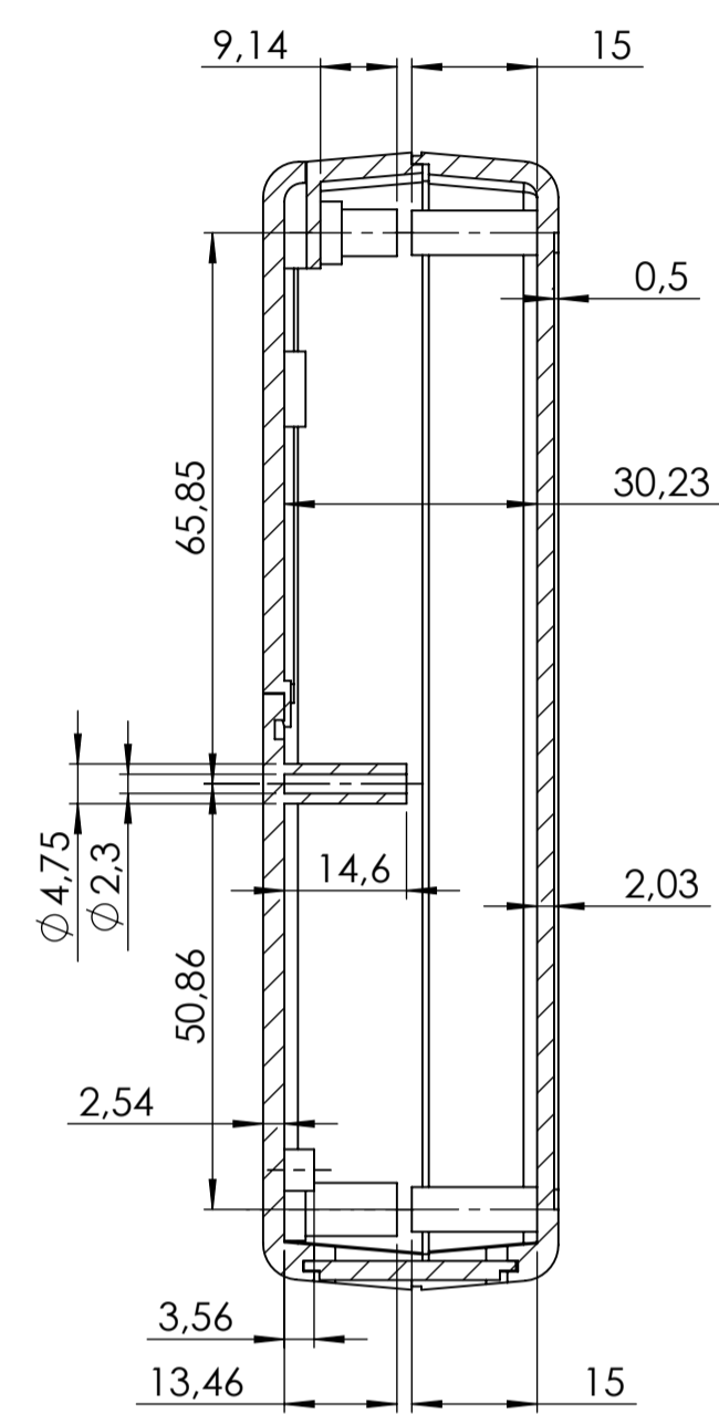
SEZIONE A-A
