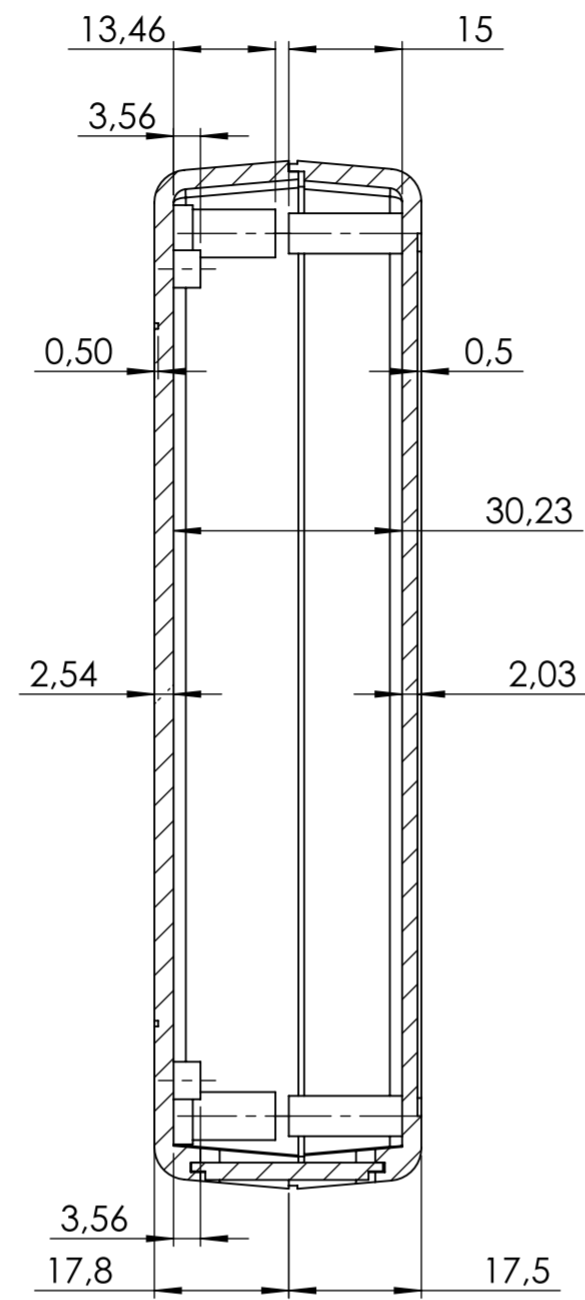
SEZIONE A-A
