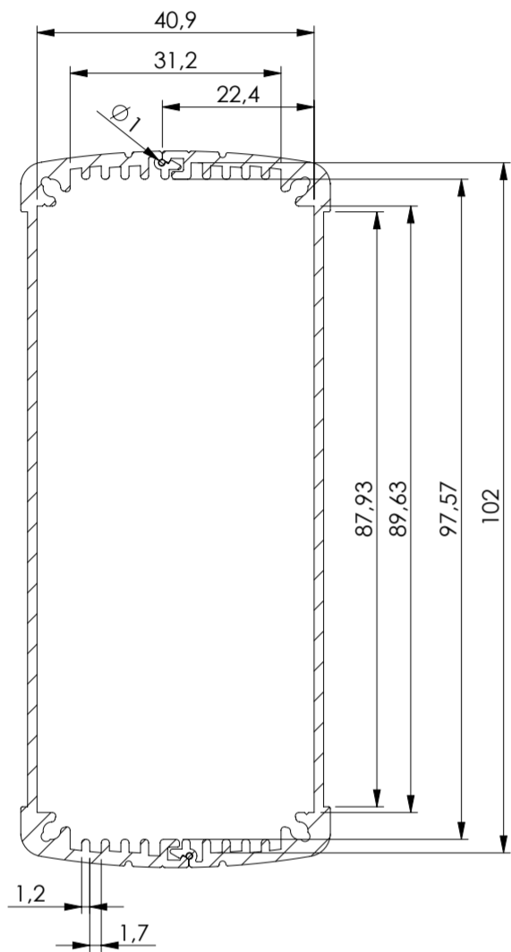
SEZIONE A-A
